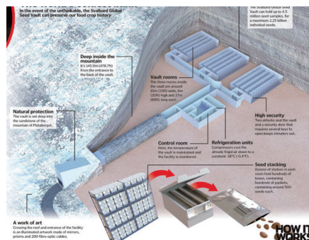
圖四：「末日種子庫」的剖面結構圖，最深處的三個房間是存放種子的庫房
